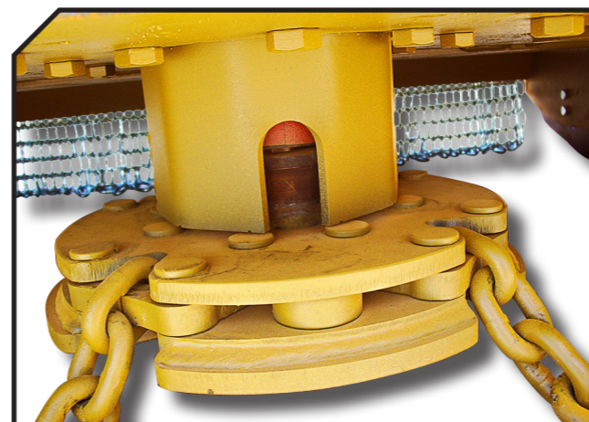
SERRAT ротор со сменными цепями
